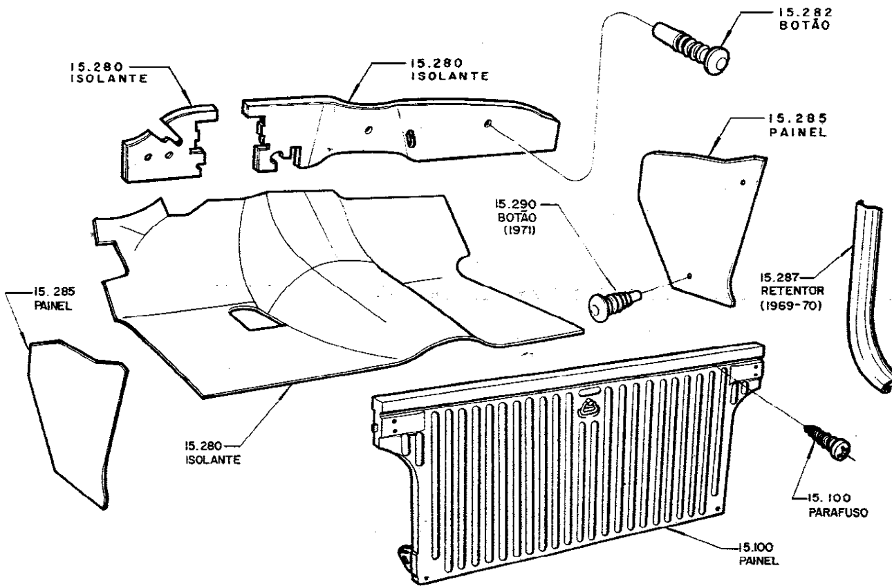
ISOLANTE DO ASSOALHO
