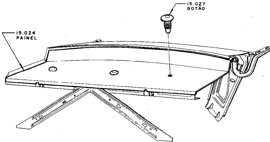
PAINEL DE ACABAMENTO TRASEIRO SUPERIOR
