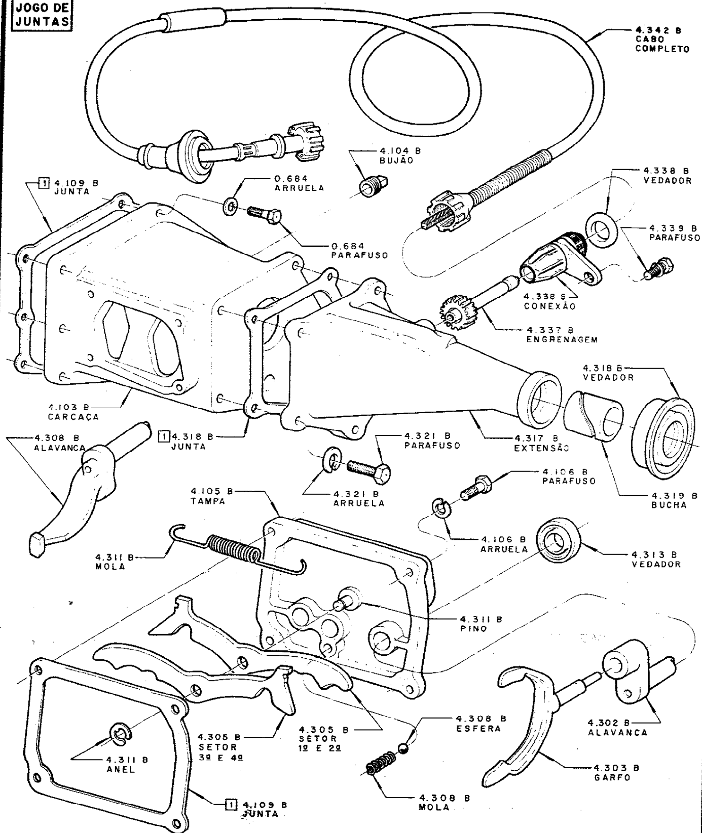
CAIXA DE MUDANÇAS — CARÇA E MECANISMO — 4 VELOCIDADES
