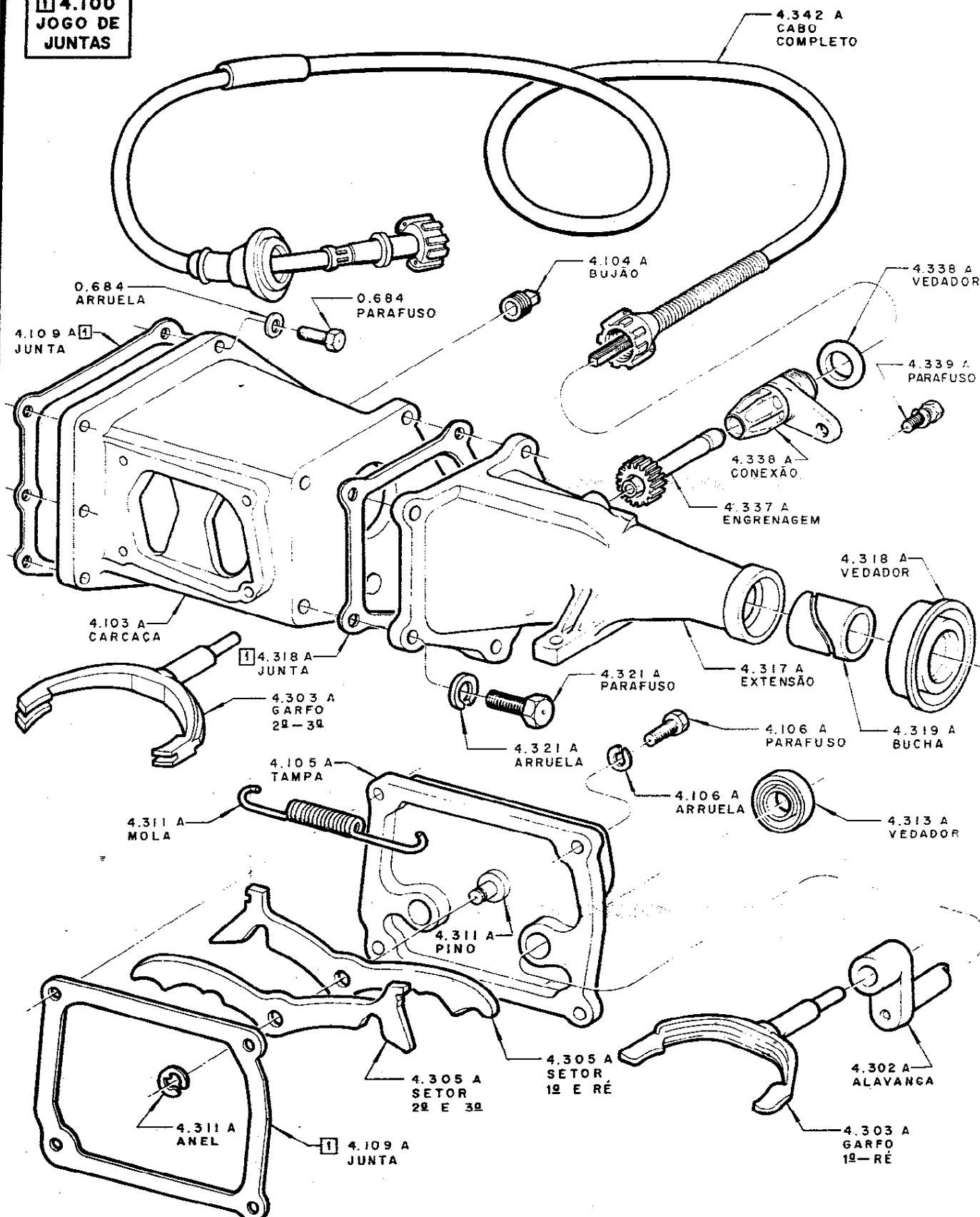
CAIXA DE MUDANÇAS — CARCAÇA E MECANISMO — 3 VELOCIDADES
