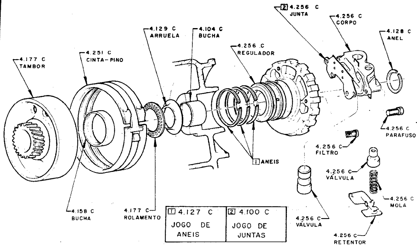
REGULADOR CENTRÍFUGO E TAMBOR DO PLANETÁRIO
