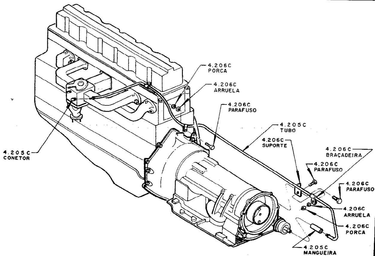
LINHA DO TUBO DE VÁCUO
