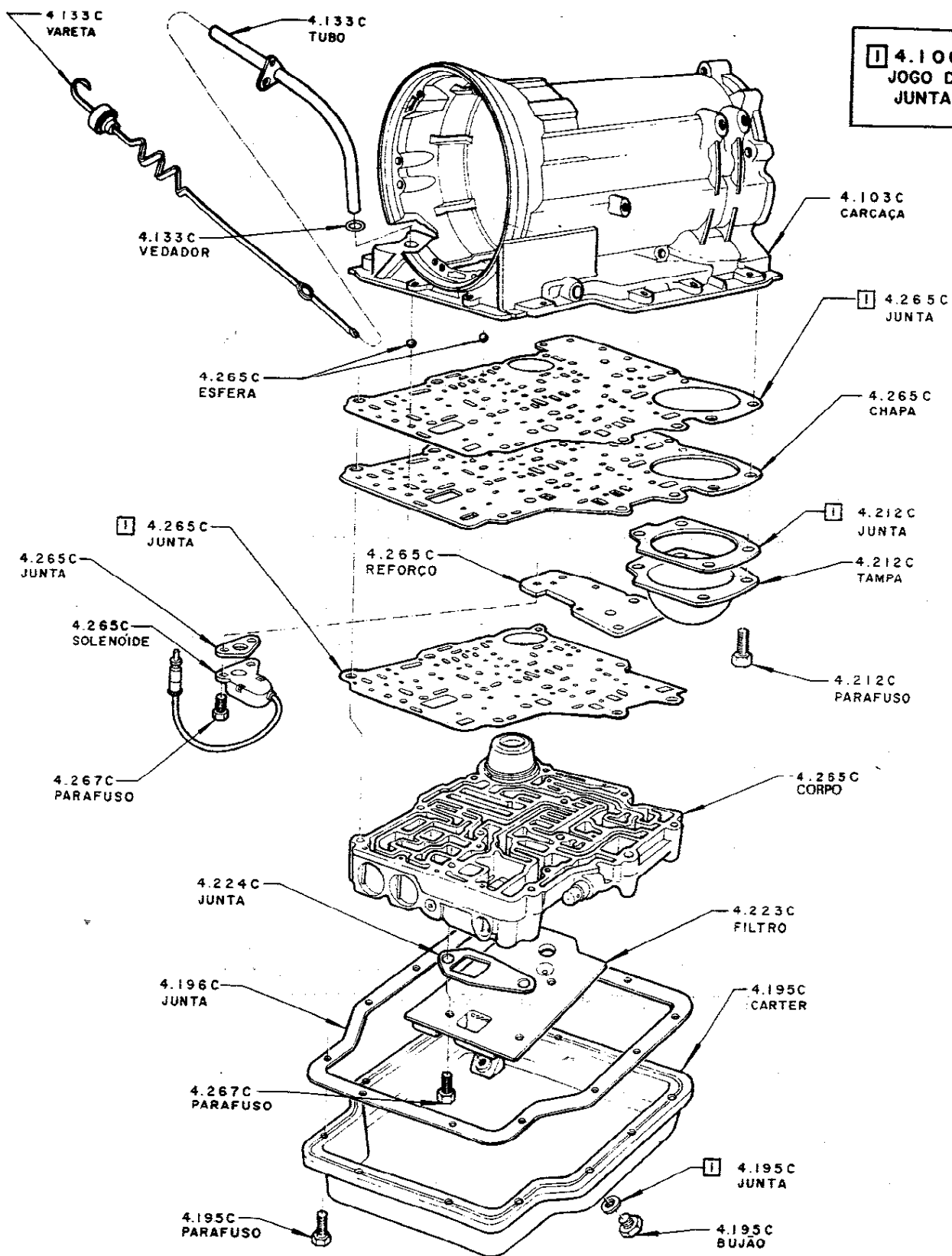
CARTER — FILTRO — JUNTAS E CHAPA DA PASSAGEM DO ÓLEO
