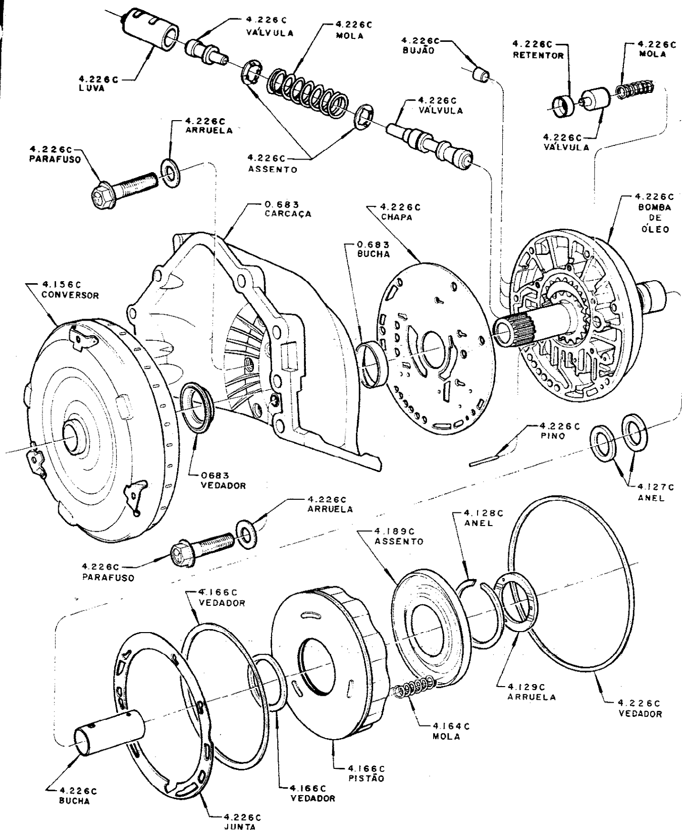
CONVERSOR E BOMBA DE ÓLEO
