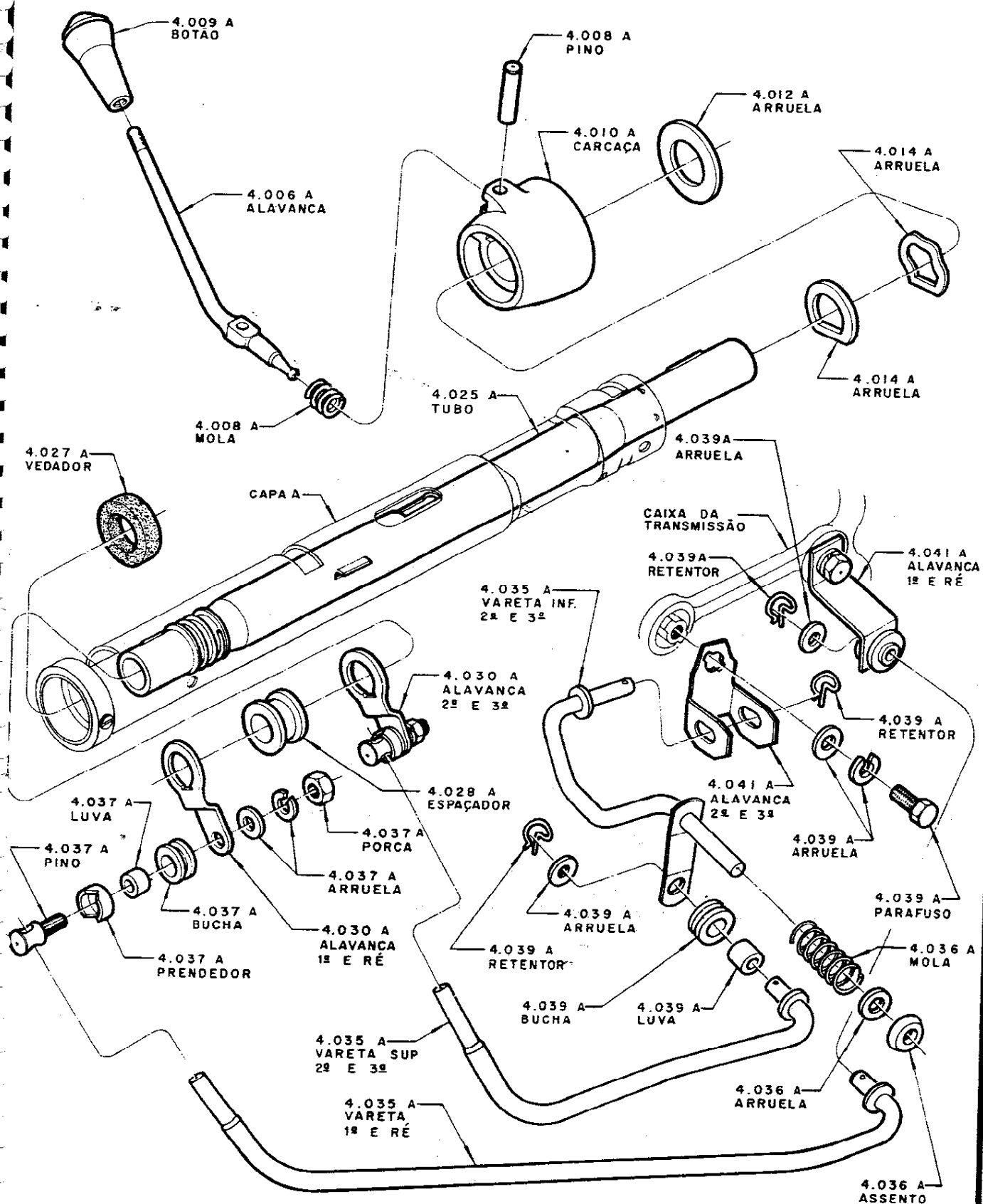
MECANISMO DA MUDANÇA - 3 VELOCIDADES
