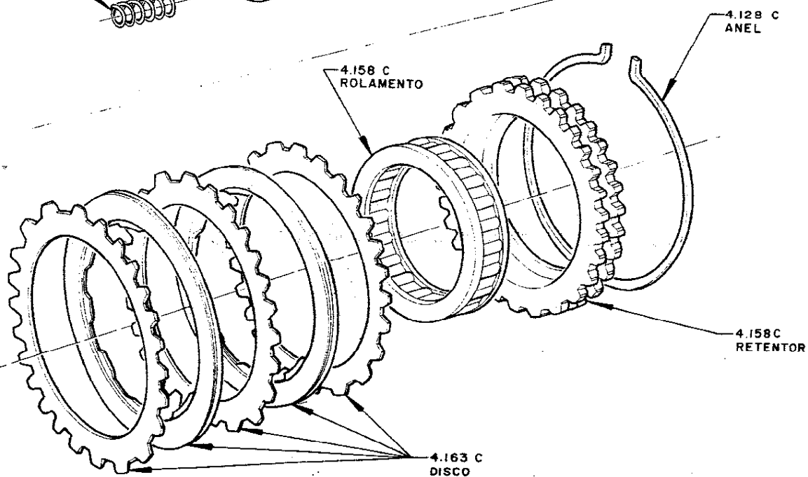
JOGO DE EMBREAGEM DA 3ª
