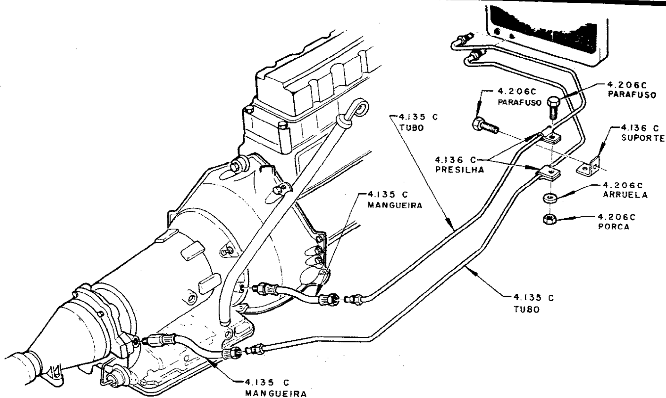
LINHA DO TUBO DE REFRIGERAÇÃO DO ÓLEO
