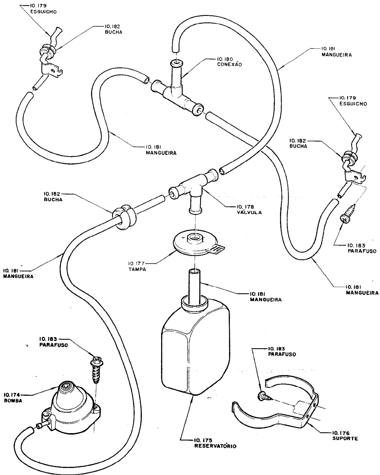
LAVADOR DO PÁRA-BRISA
