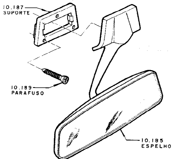
ESPELHO RETROVISOR INTERNO
