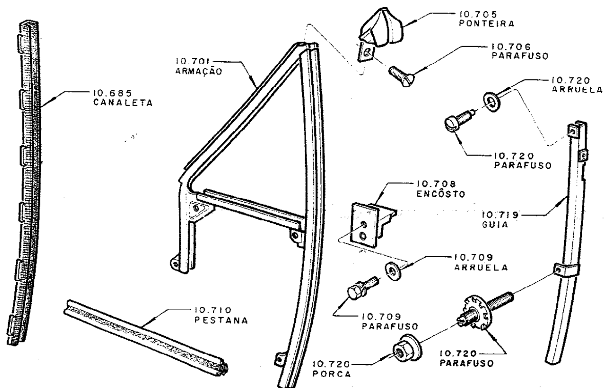
ARMAÇÃO DA JANELA DA PORTA — 2 PORTAS
