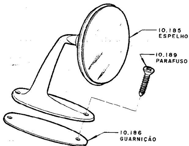
ESPELHO RETROVISOR EXTERNO
