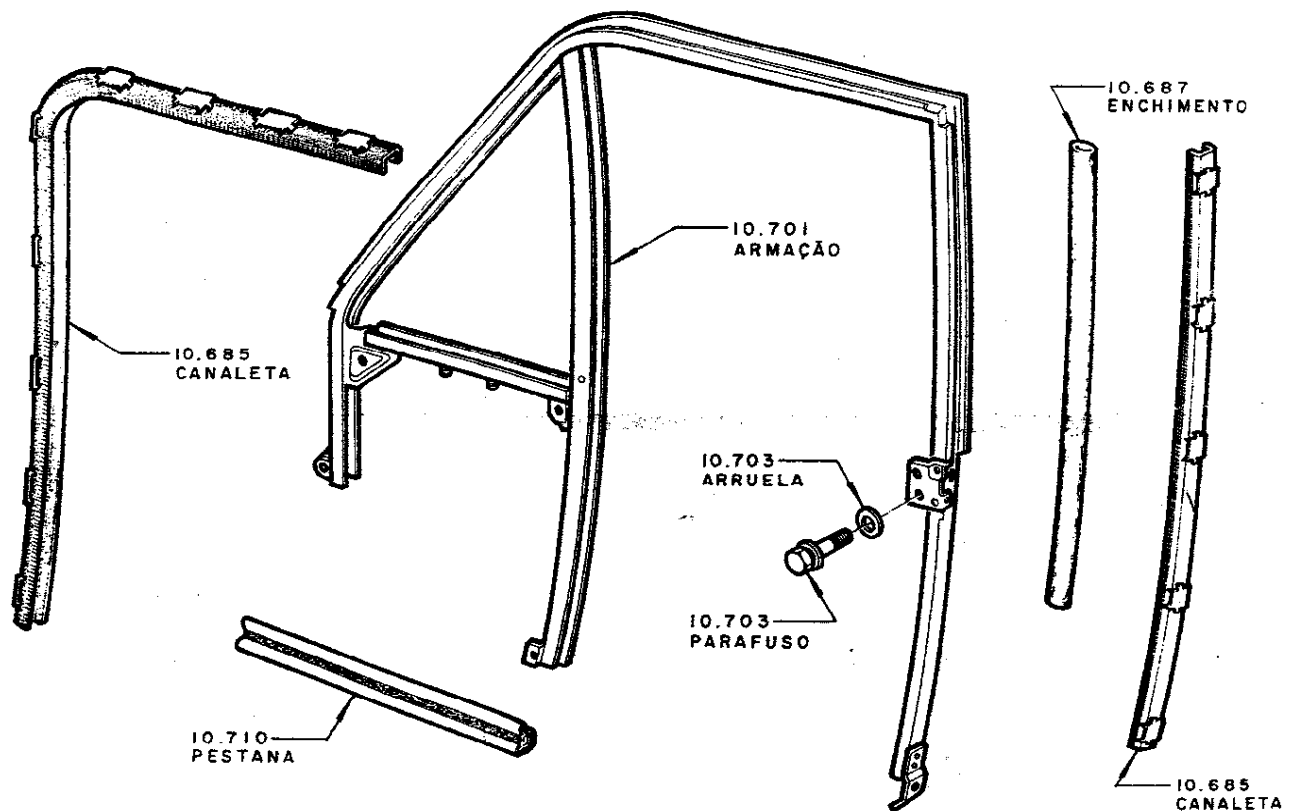
ARMAÇÃO DA JANELA DA PORTA DIANTEIRA — 4 PORTAS
