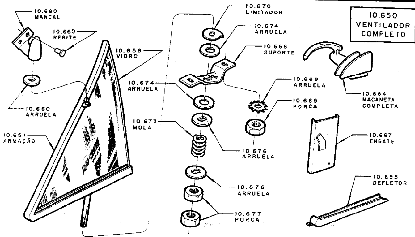
VENTILADOR DA PORTA
