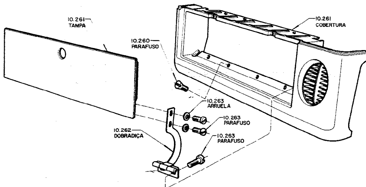
CAIXA E TAMPA DO PORTA - LUVAS (1969-74)
