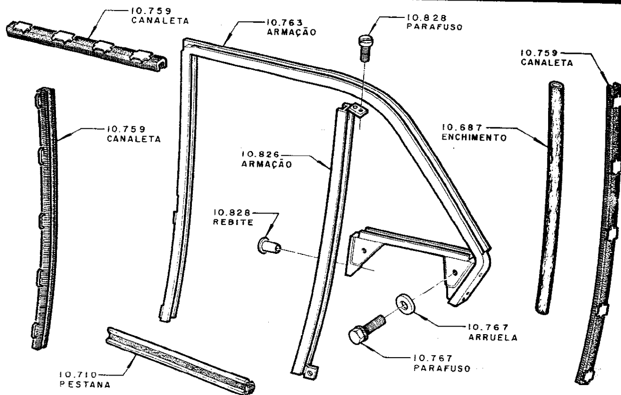
ARMAÇÃO DA JANELA DA PORTA TRASEIRA
