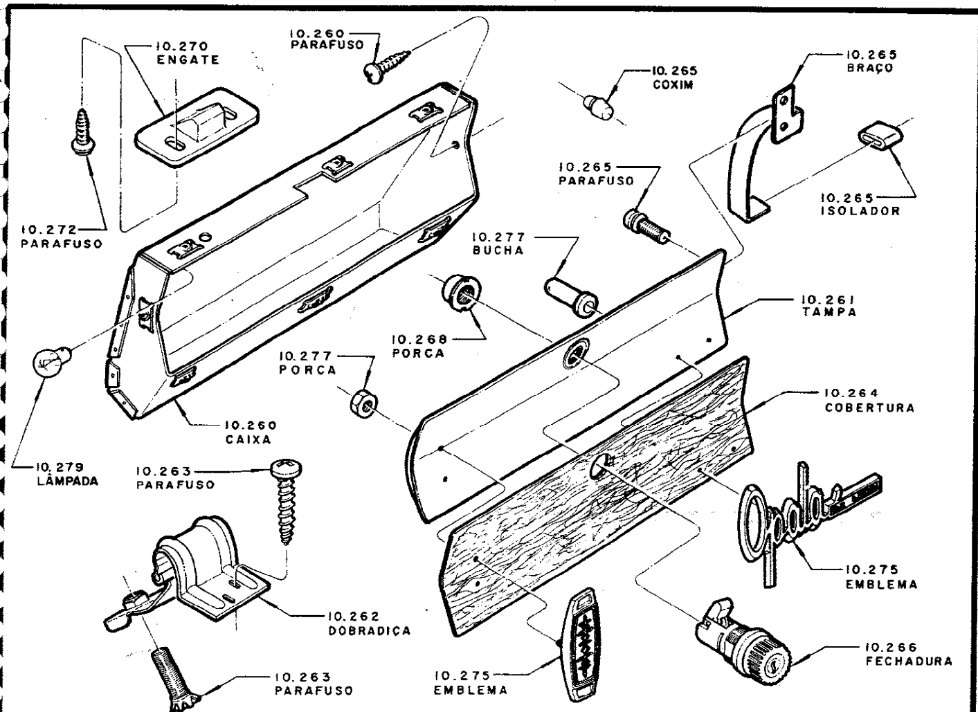
CAIXA E TAMPA DO PORTA - LUVAS (1969-74)
