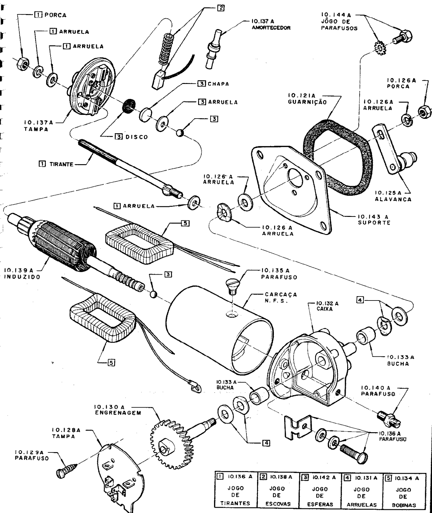
MOTOR DO LIMPADOR DO PÁRA-BRISA - "ARNO"
