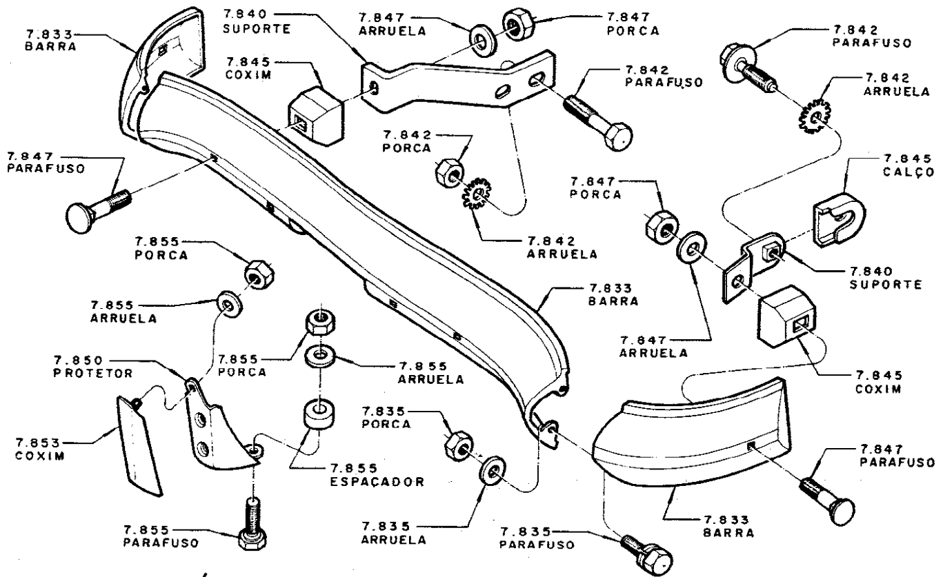
PÁRA-CHOQUE DIANTEIRO — 7.831
