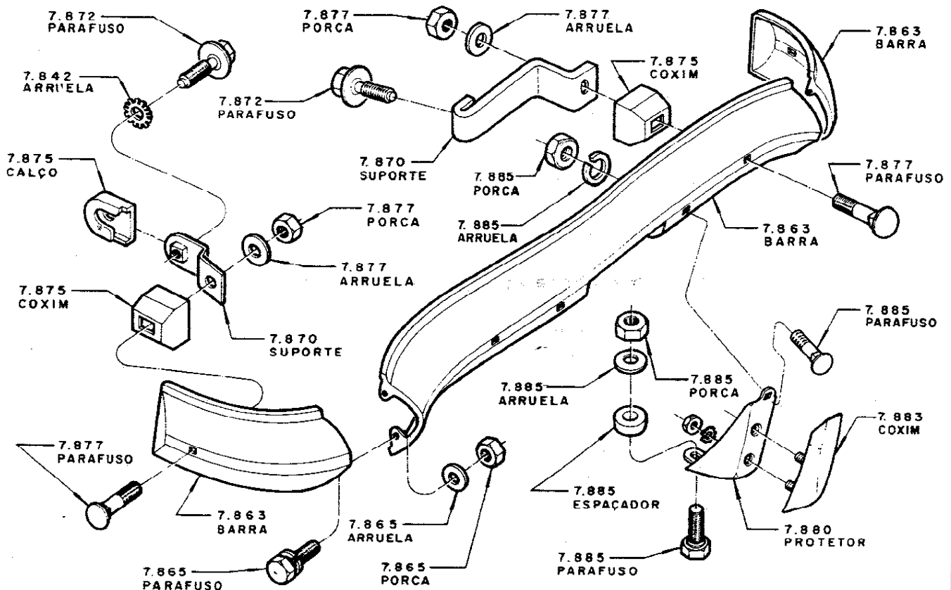
PÁRA-CHOQUE TRASEIRO — 7.861
