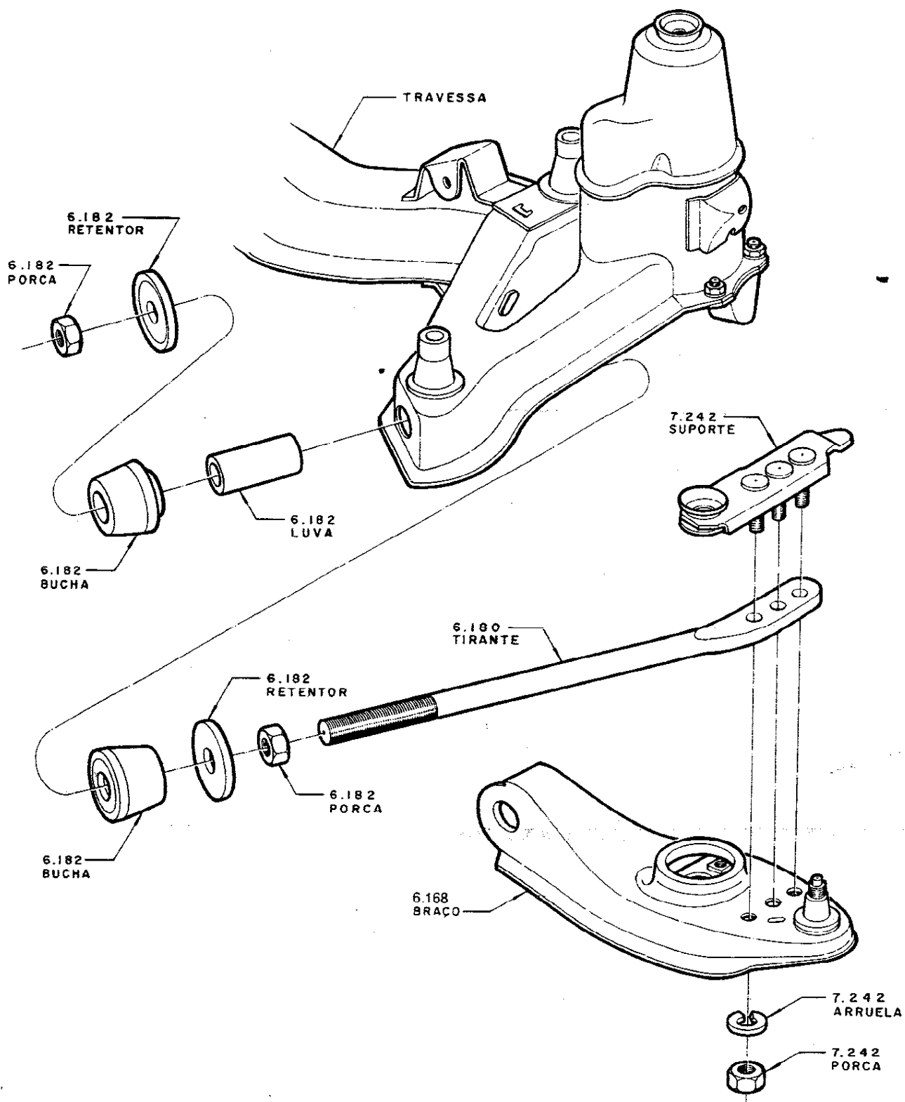
TIRANTE SUJEITADOR DO BRAÇO DE CONTRÔLE
