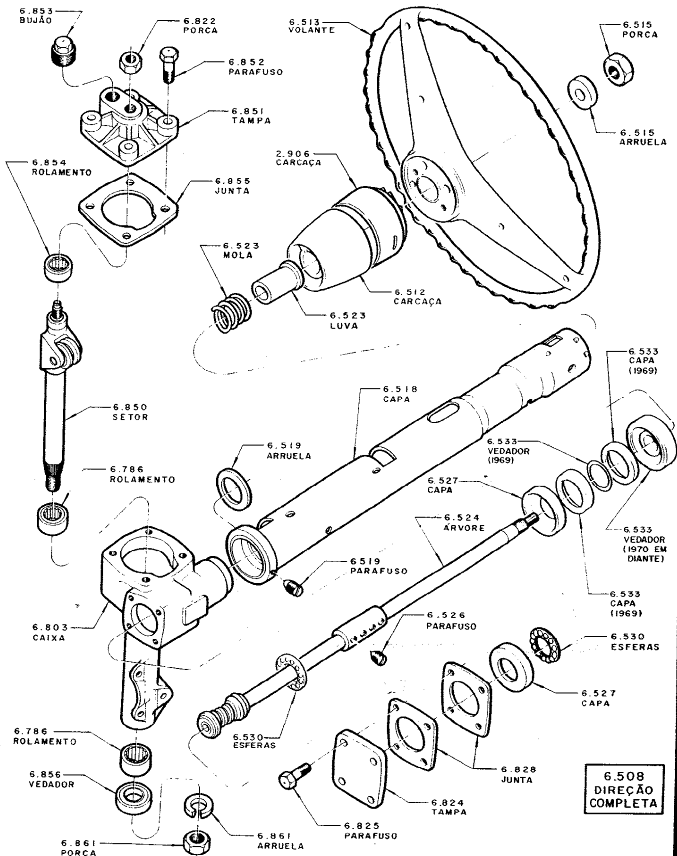
MECANISMO DA DIREÇÃO
