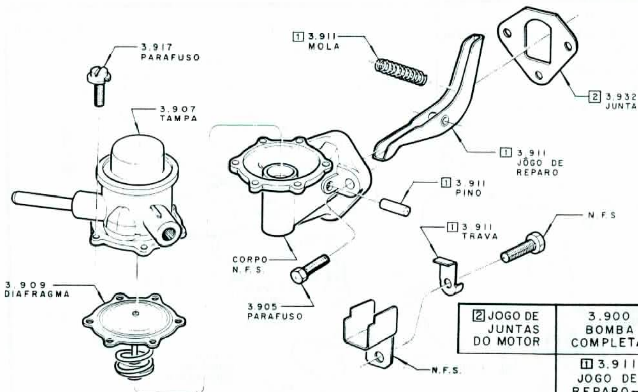
BOMBA DE GASOLINA "BROSOL"
