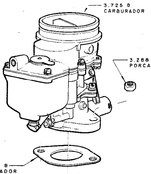
FIXAÇÃO DO CARBURADOR DFV
