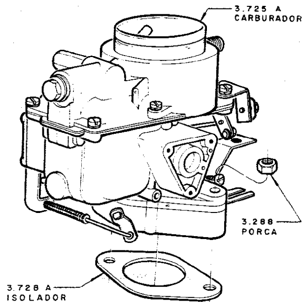
FIXAÇÃO DO CARBURADOR SOLEX
