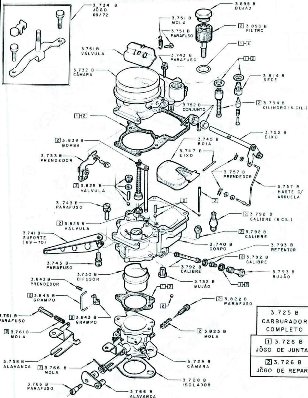
CARBURADOR SIMPLES "DFV"
