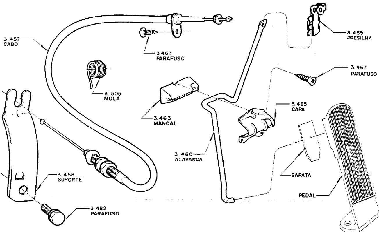
PEDAL DO ACELERADOR E CONTRÔLES - 3º TIPO
