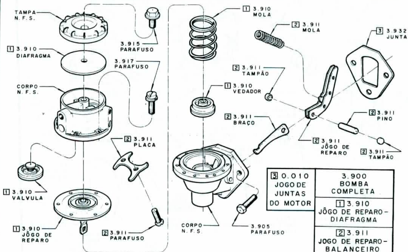
BOMBA DE GASOLINA "GM-DFV"
