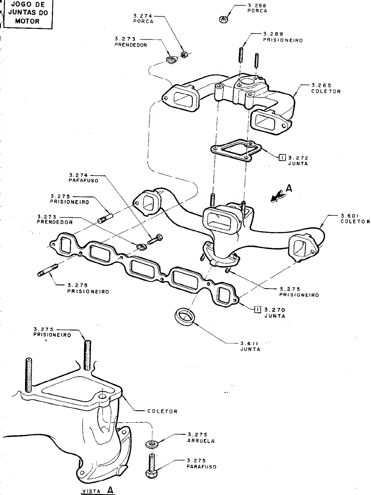
COLETORES - 4 CILINDROS
