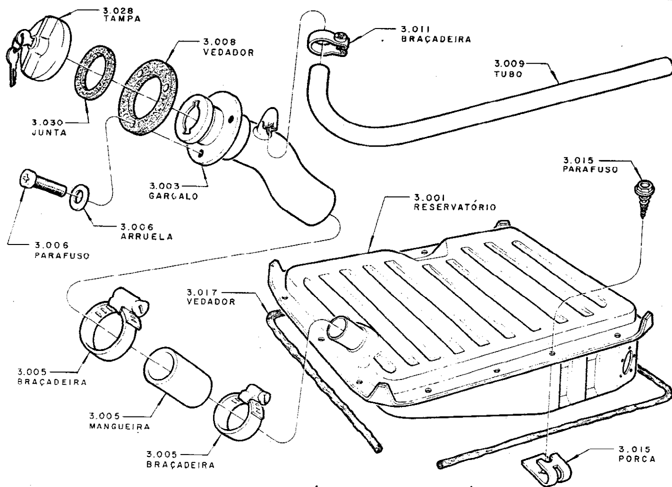
1971-1975-RESERVATÓRIO DE COMBUSTÍVEL
