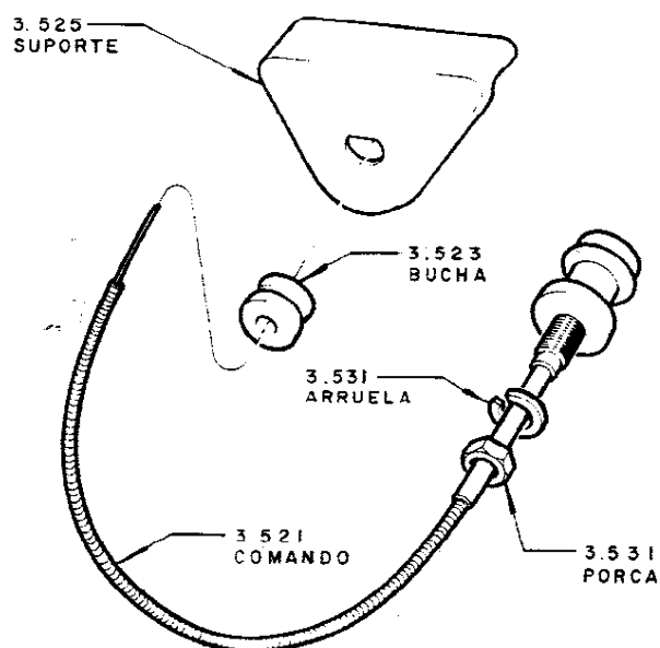
COMANDO MANUAL DO ABAFADOR
