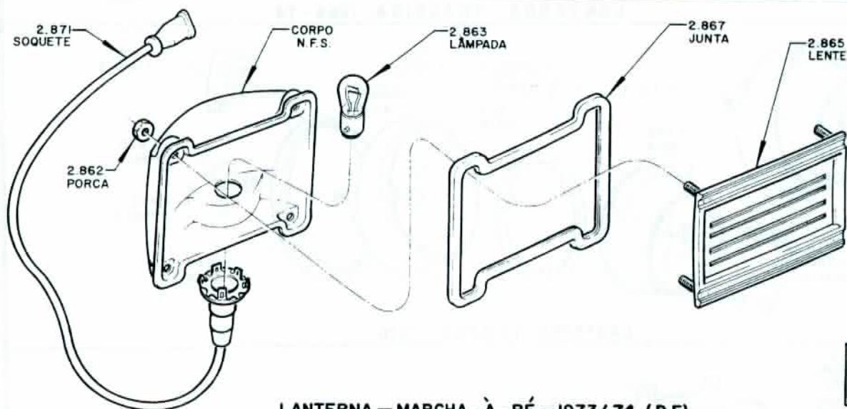
LANTERNA — MARCHA - À - RÉ — 1973/ 74 (D.F.)
