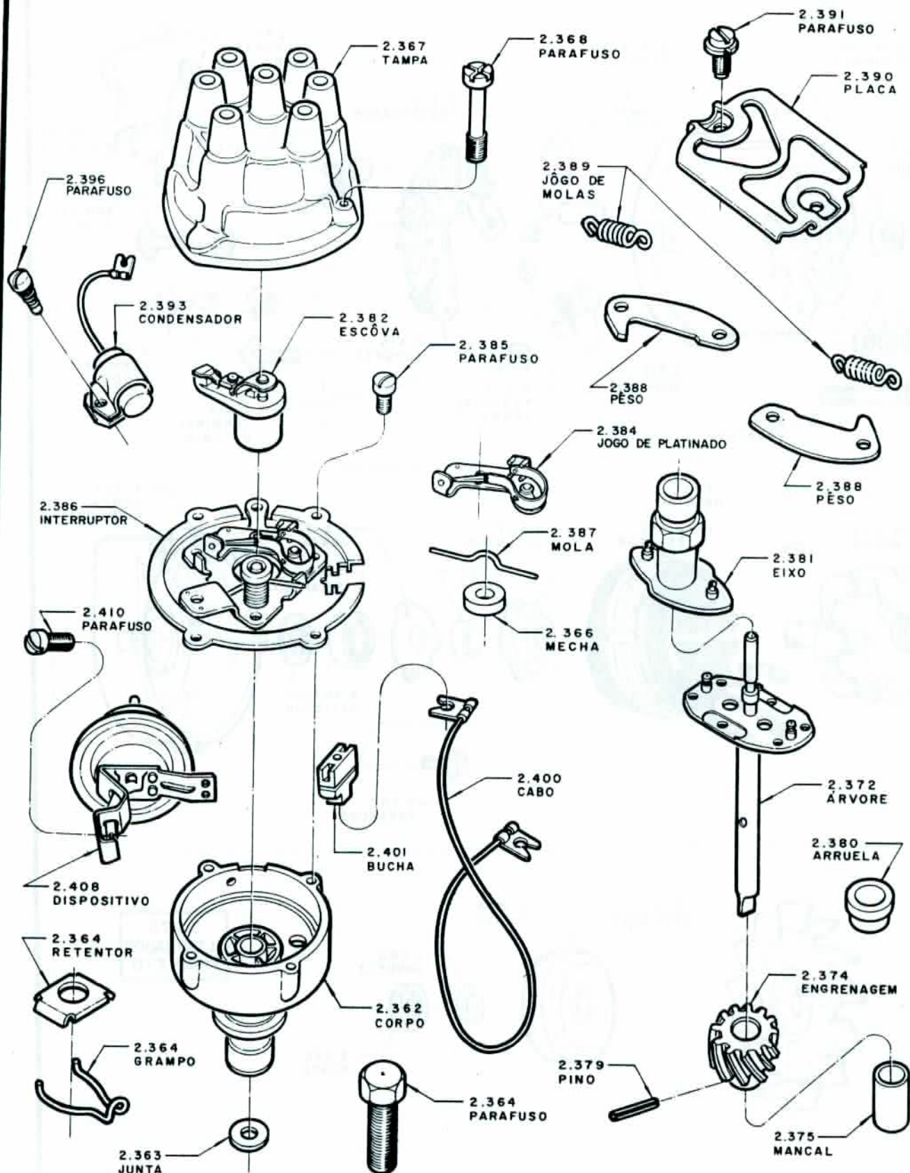
Gr. 2.361 - DISTRIBUIDOR DE IGNIÇÃO (6 CILINDROS MOSTRADO)
