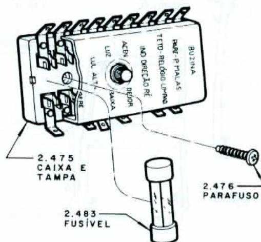
CAIXA DE FUSÍVEIS — 1972/73
