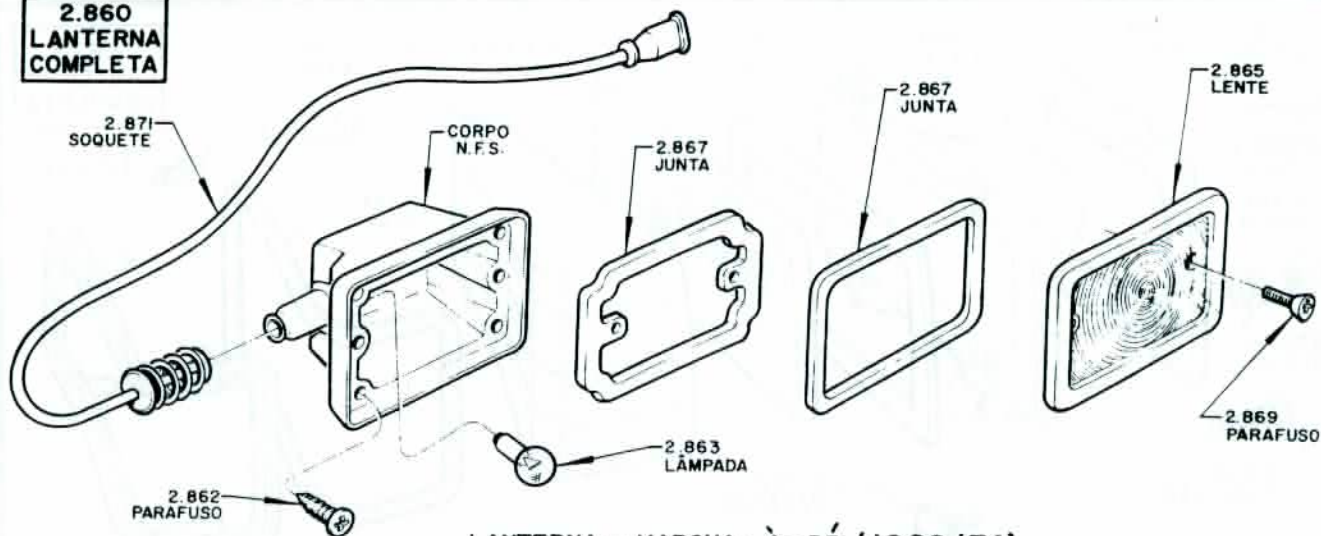
LANTERNA — MARCHA - À - RÉ (1969/74)
