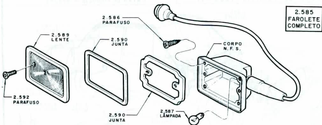
FAROLETE DE ESTACIONAMENTO 69/72
