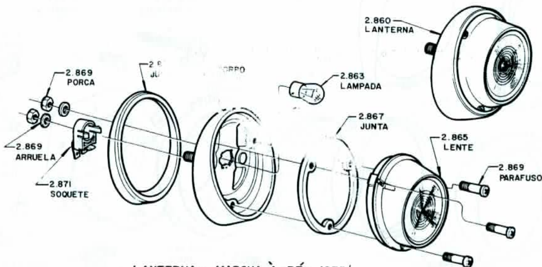
LANTERNA - MARCHA-À- RÉ - 1975/
