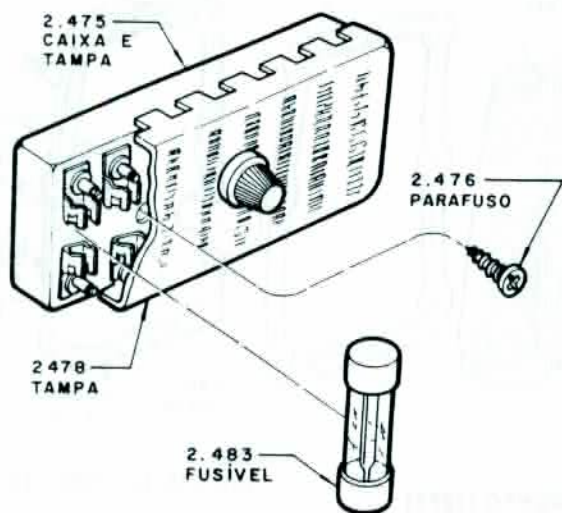
CAIXA DE FUSÍVEIS — 1969 — 71
