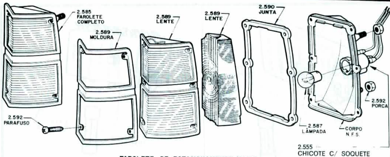
FAROLETE DE ESTACIONAMENTO (1975)
