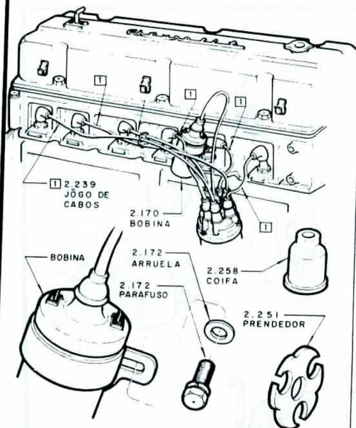
BOBINA E CABOS DAS VELAS
