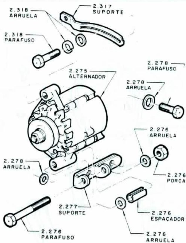
FIXAÇÃO DO ALTERNADOR
