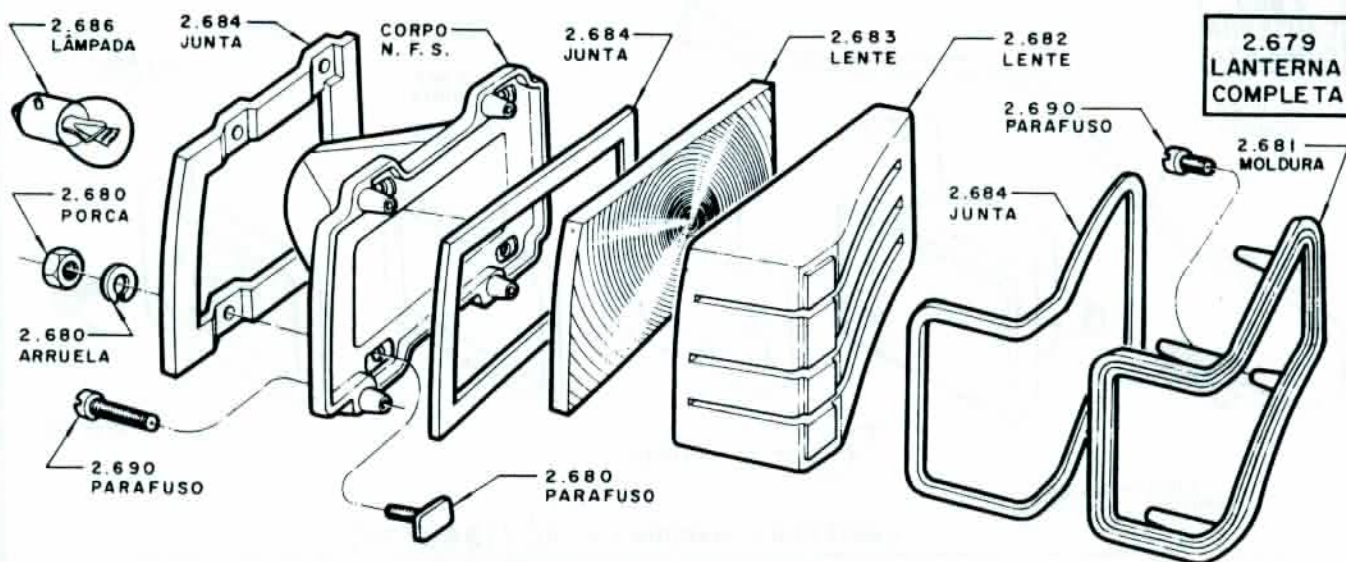
LANTERNA TRASEIRA- 1969- 74
