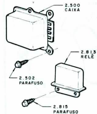
CAIXA DO REGULADOR — RELÊ DA BUZINA
