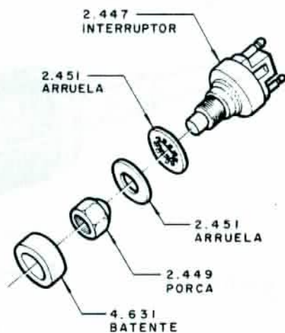
INTERRUPTOR DO "PARE"
