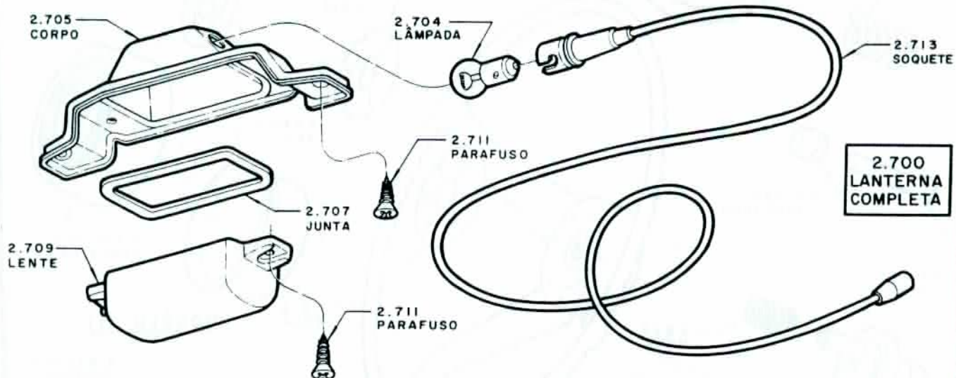
LANTERNA DA LICENÇA
