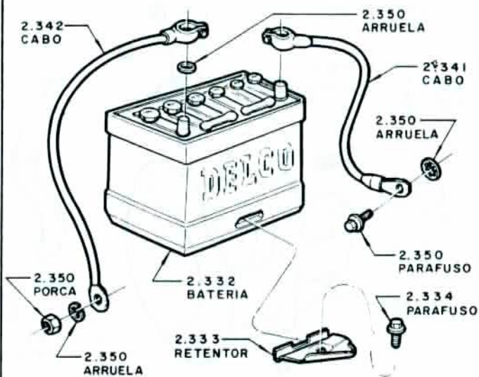
BATERIA E CABOS
