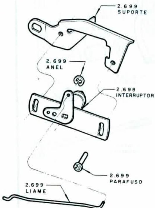
INTERRUPTOR - MARCHA A RÉ - 4 VELOCIDADES
