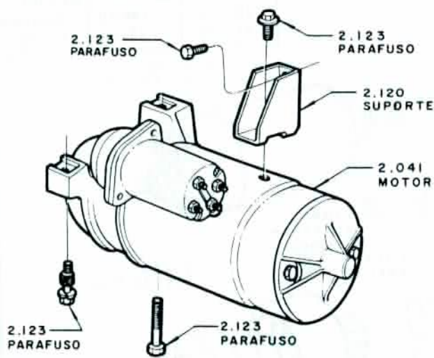
FIXAÇÃO DO MOTOR DE PARTIDA
