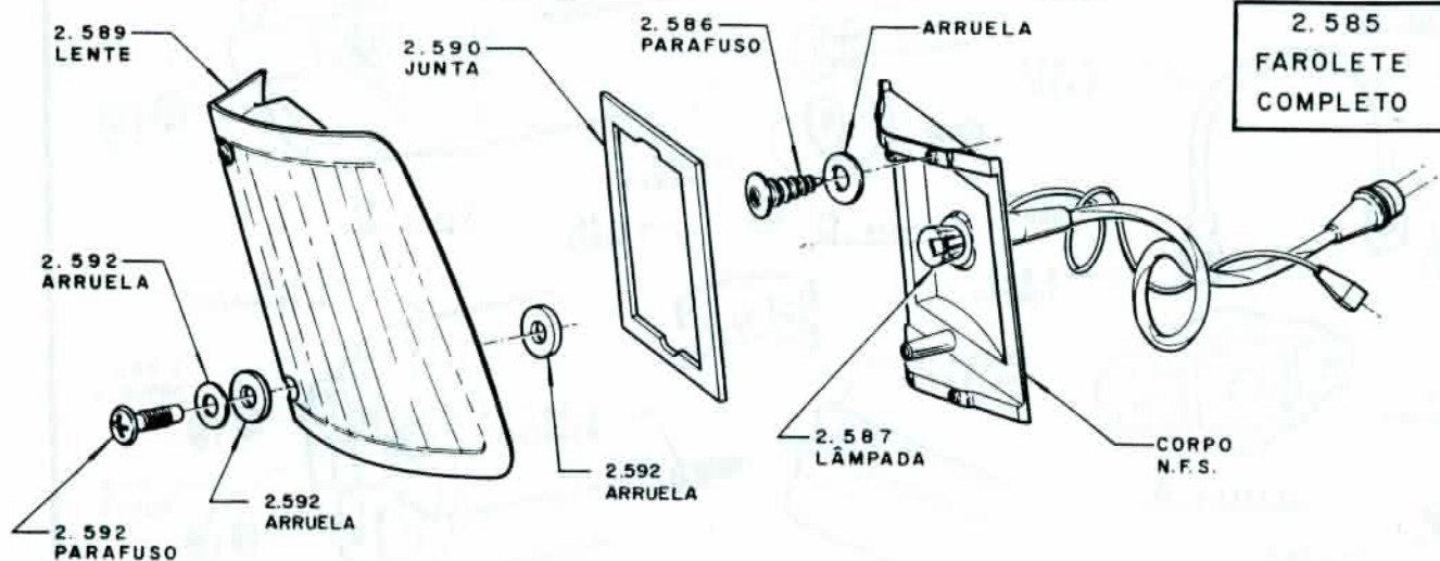
FAROLETE DE ESTACIONAMENTO 73/74
