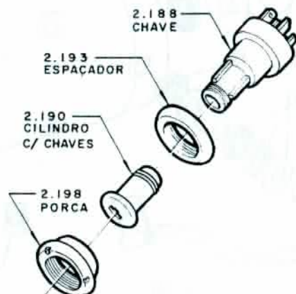
INTERRUPTOR DO "PARE"
