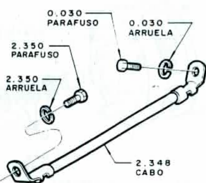
COMUTADOR DA LUZ ALTA E BAIXA
