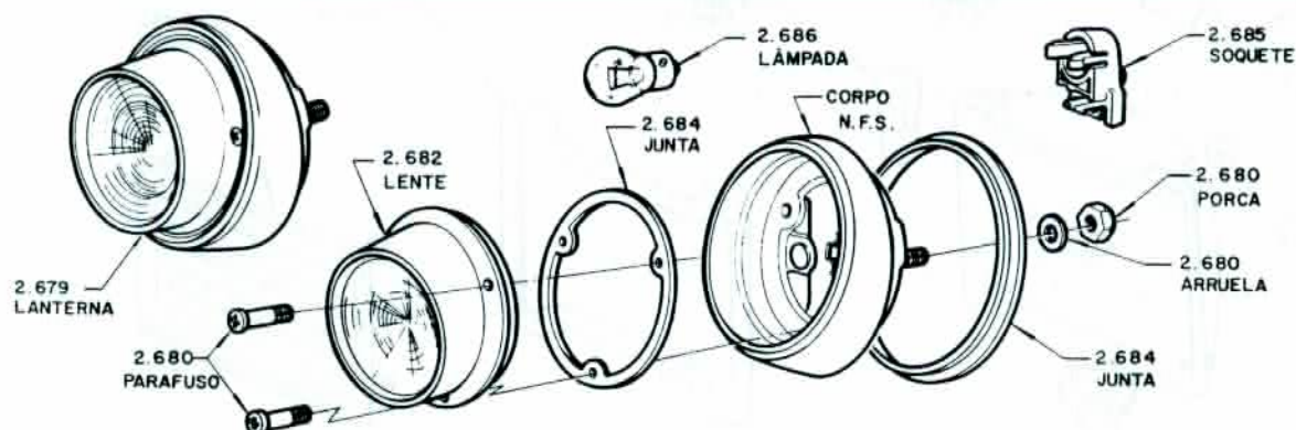
LANTERNA TRASEIRA- 1975
