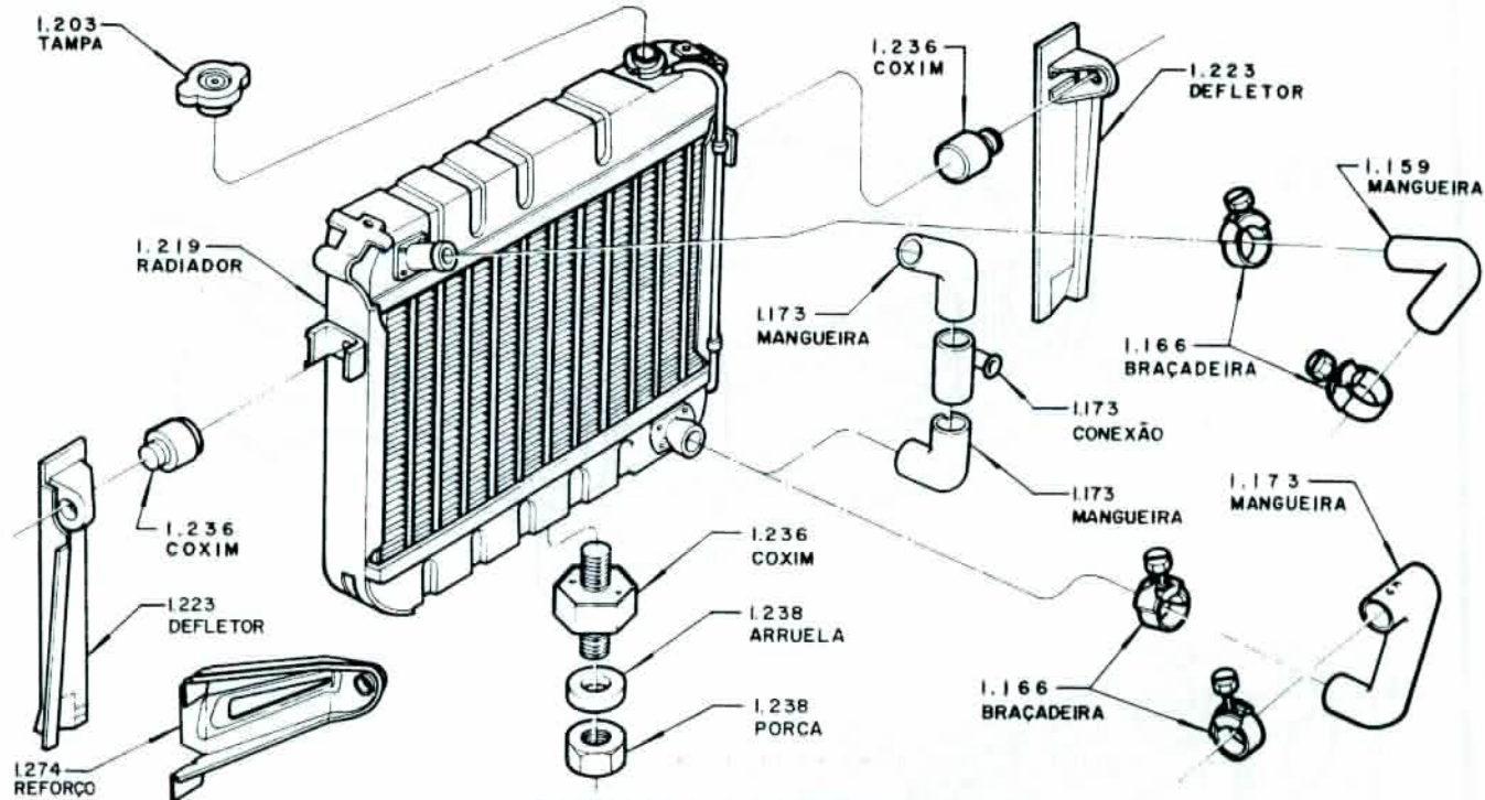
RADIADOR — 4 CILINDROS
