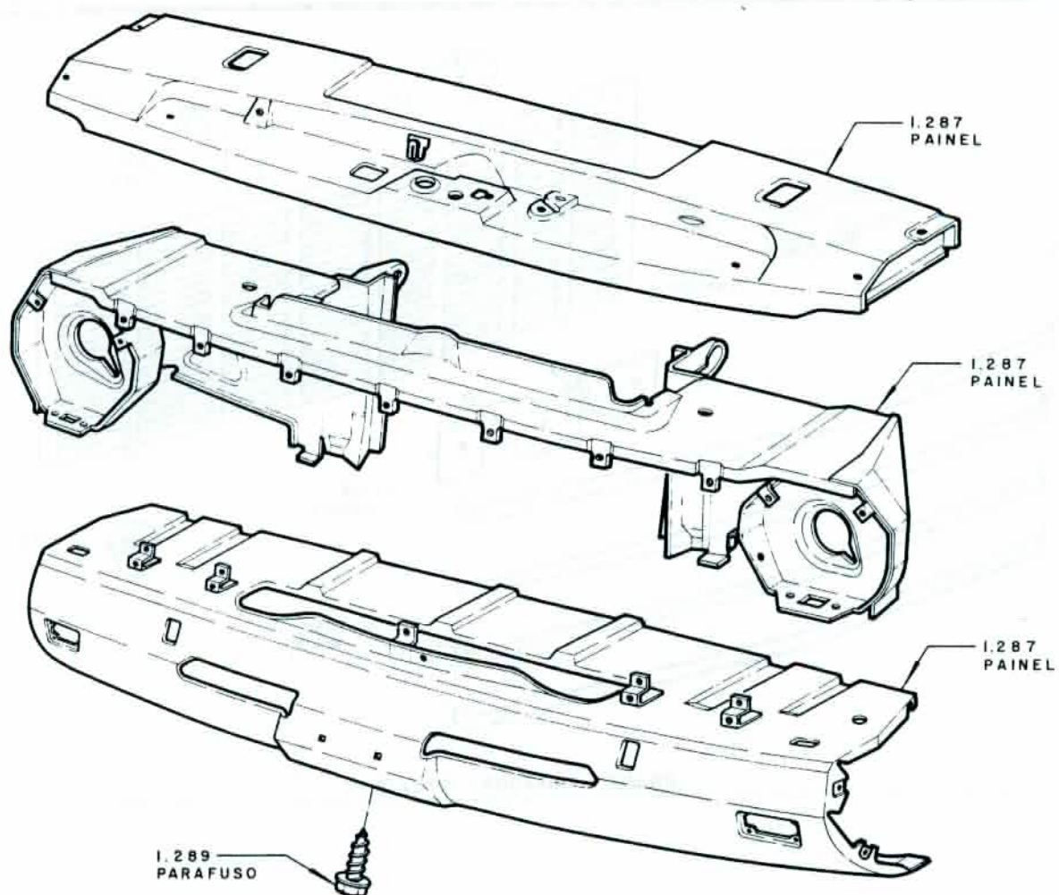
PAINEIS DIANTEIROS 69/74
