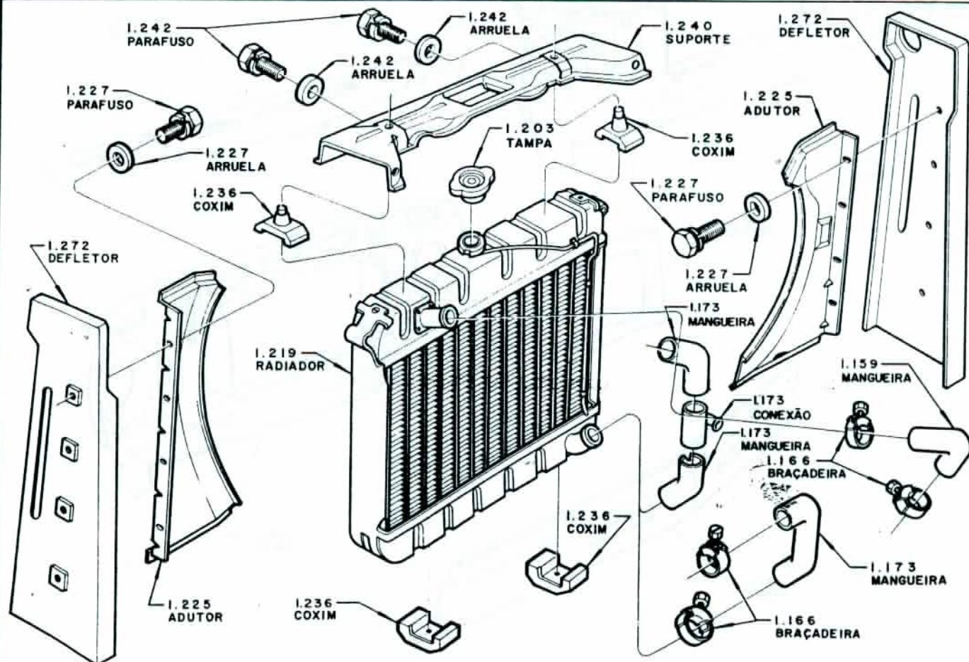
RADIADOR — 4 CILINDROS
