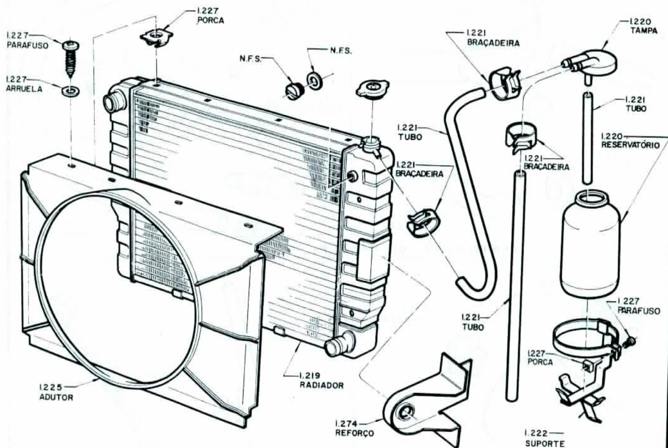
RADIADOR - 6 CILINDROS (1975/ )
