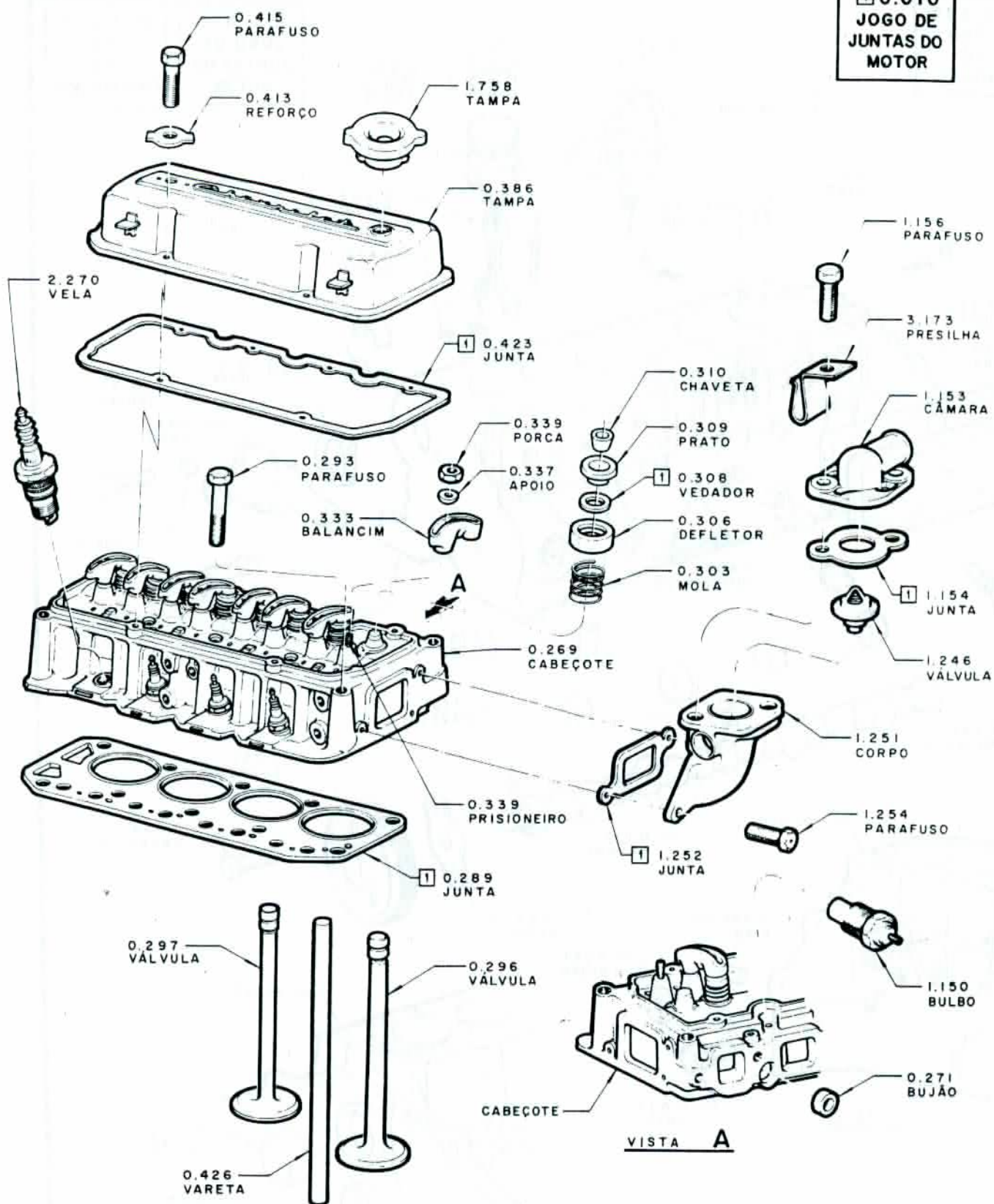
CABEÇOTE DOS CILINDROS E TAMPA DO CÁRTER — 4 CILINDROS
