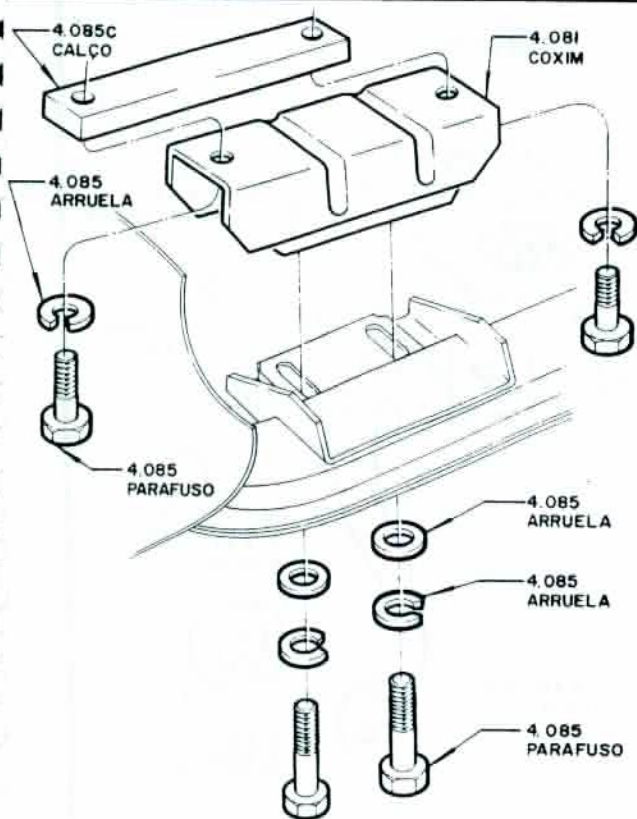
MONTAGEM CENTRAL TRASEIRA DO MOTOR
