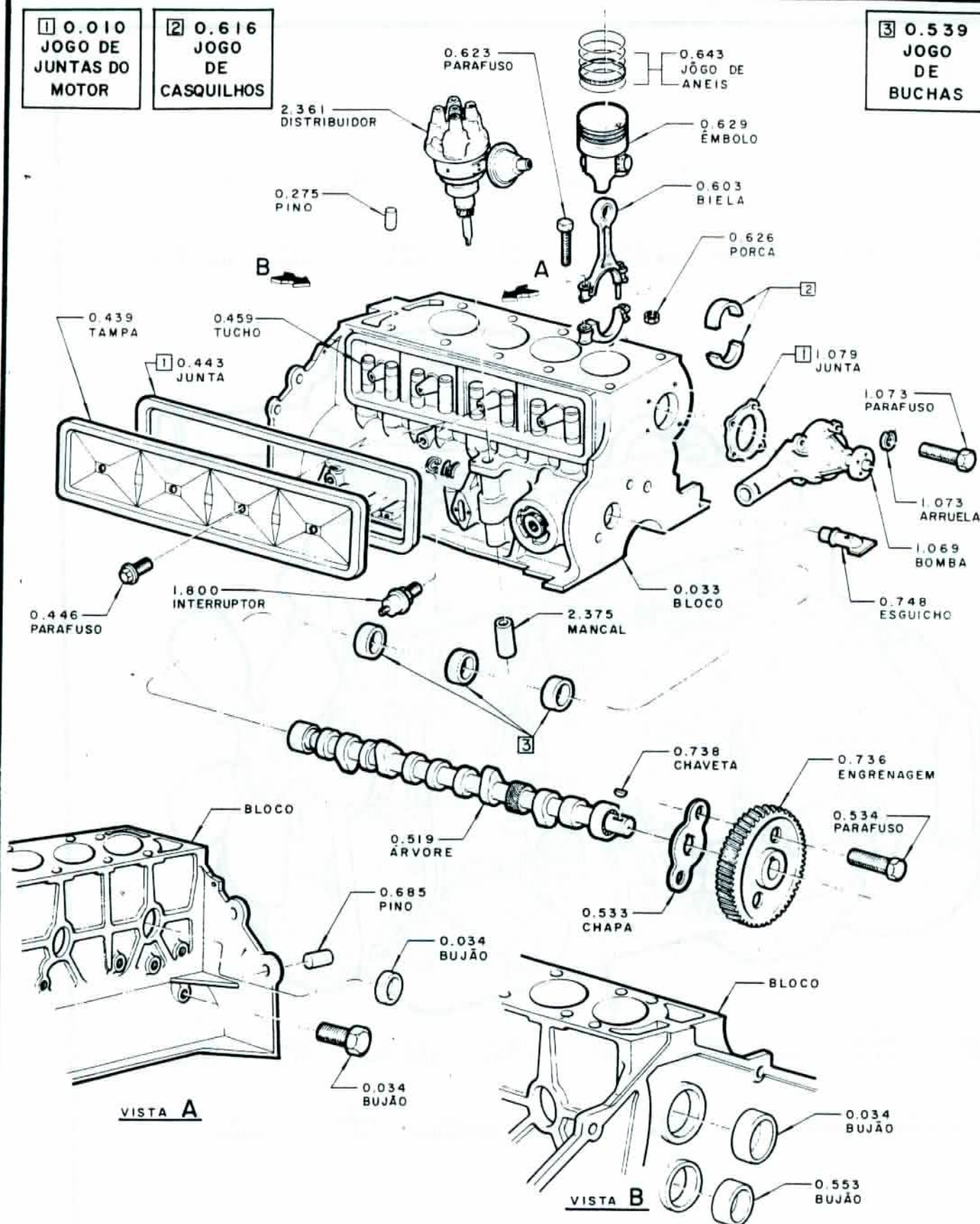
BLOCO DOS CILINDROS E ÁRVORE DE COMANDO DAS VALVULAS — 4 CILINDROS
