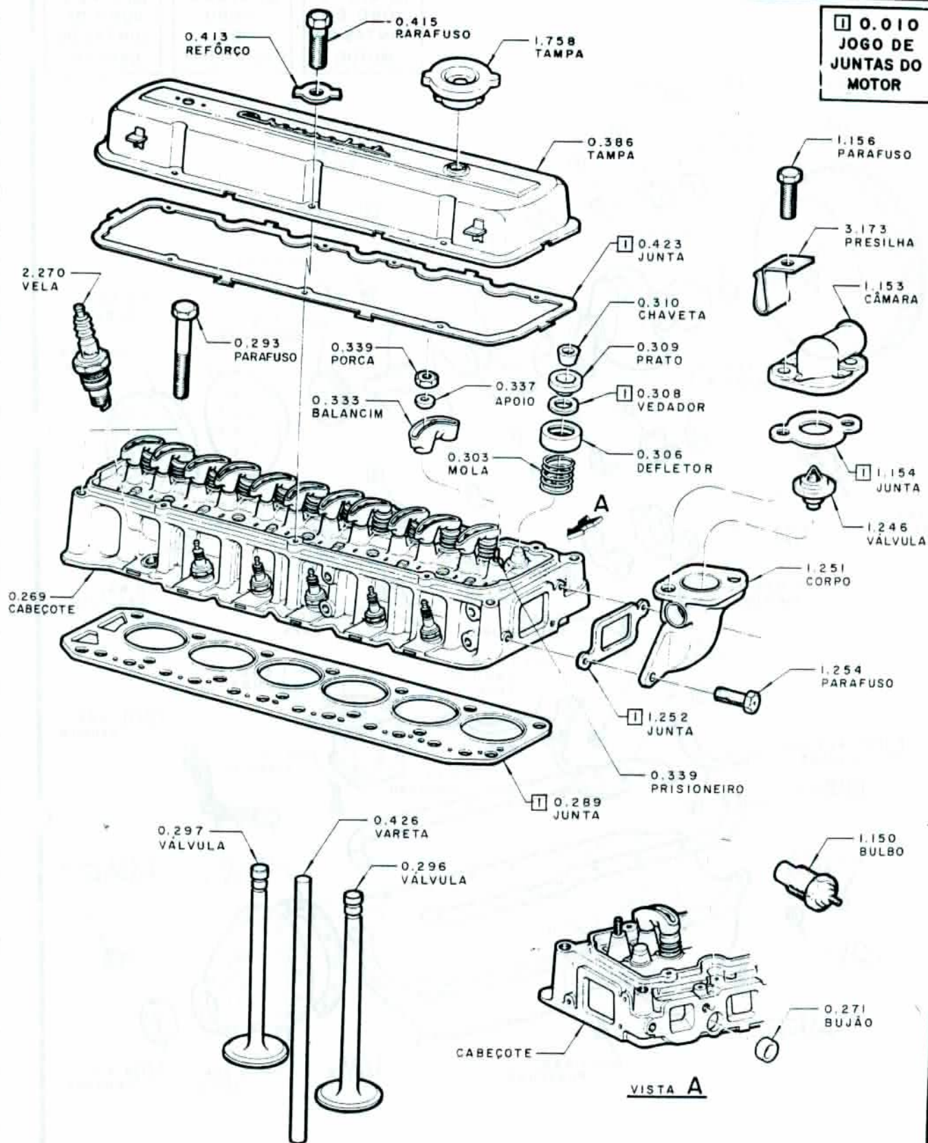
CABEÇOTE DOS CILINDROS E TAMPA DO CÂRTER — 6 CILINDROS
