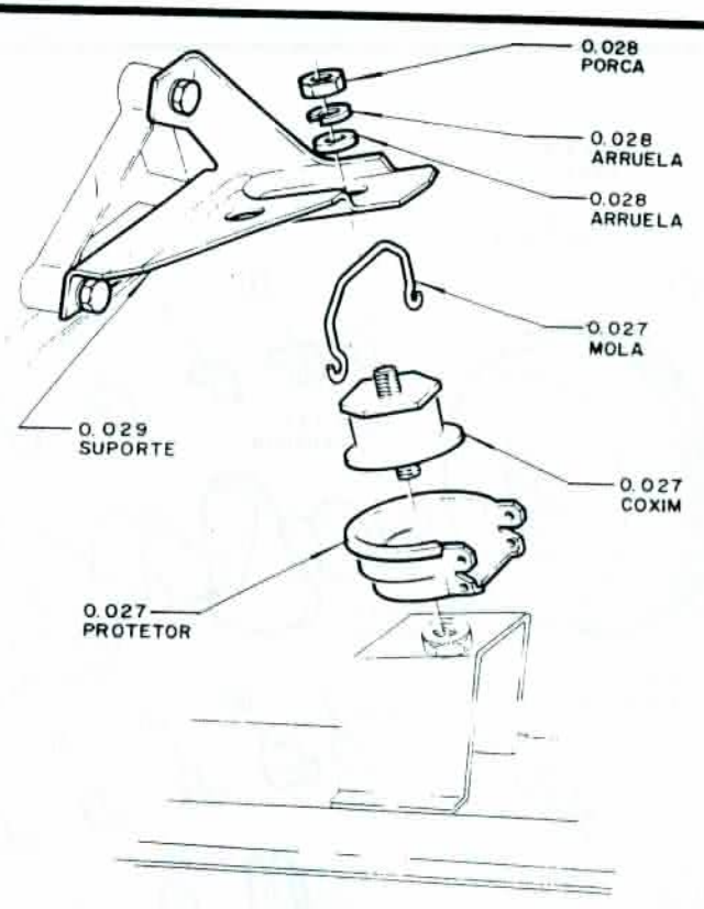
MONTAGEM DIANTEIRA DO MOTOR - 4 CIL. 74
