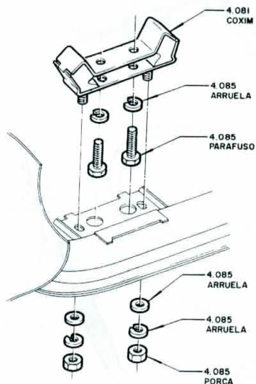
MONTAGEM CENTRAL TRASEIRA DO MOTOR-74-4 CIL
