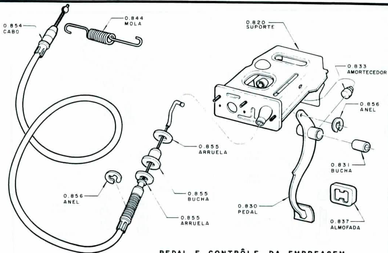
PEDAL E CONTRÔLE DA EMBREAGEM
