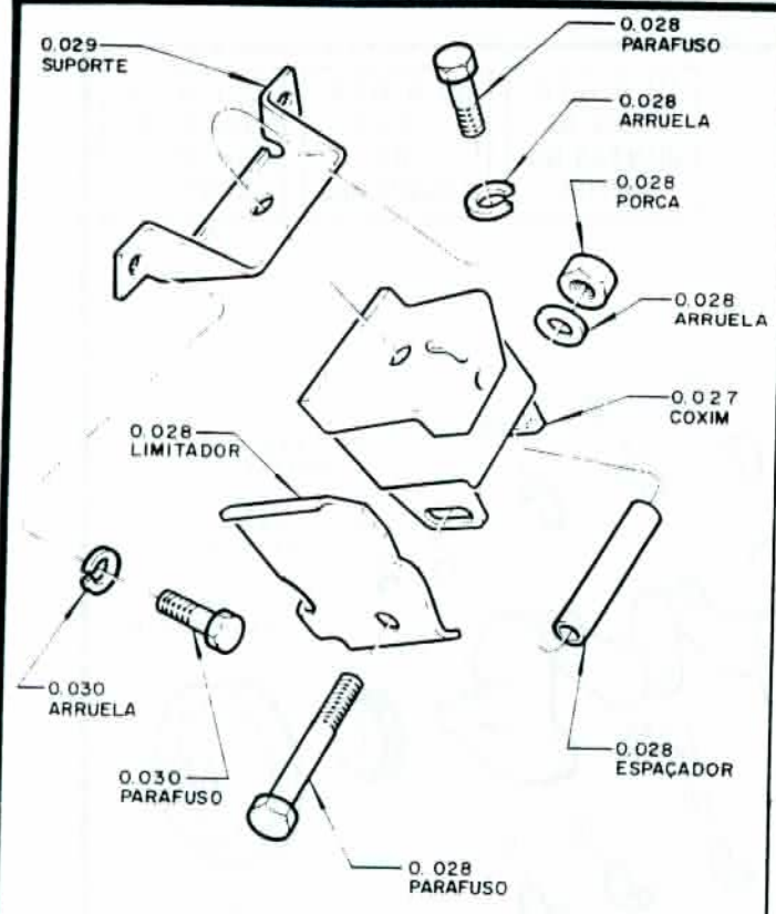
MONTAGEM DIANTEIRA DO MOTOR - 4 CIL. 69-73
