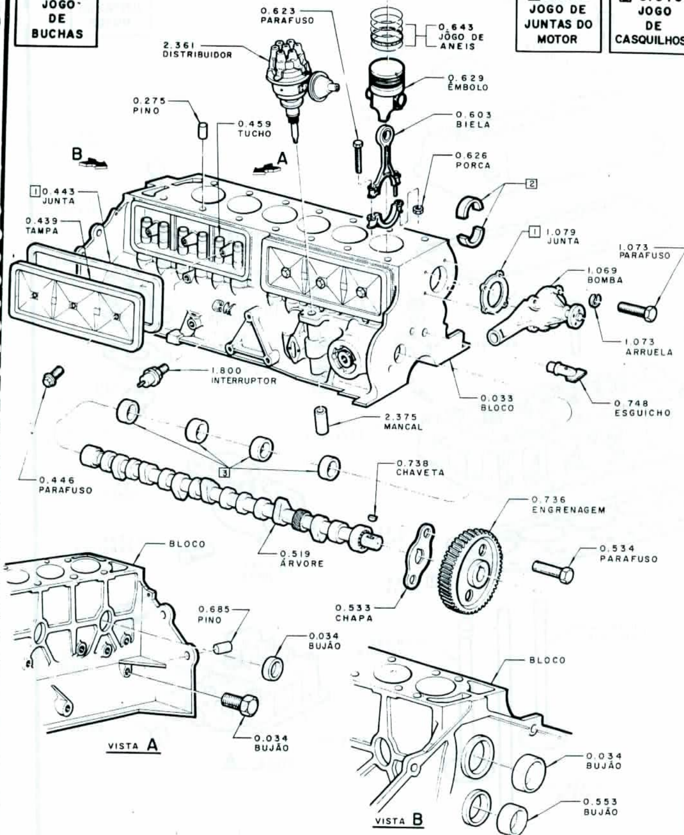
BLOCO DOS CILINDROS E ÁRVORE DE COMANDO DAS VALVULAS - 6 CILINDROS
