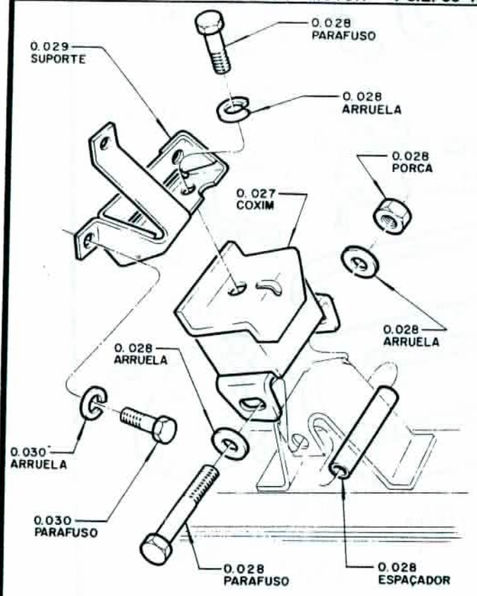
MONTAGEM DIANTEIRA DO MOTOR - 6 CIL.
