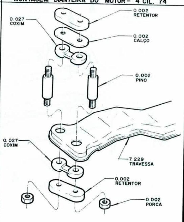
MONTAGEM LATERAL TRASEIRA DO MOTOR
